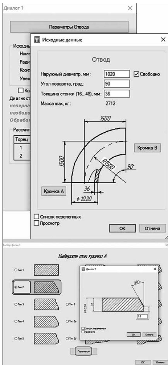
Рис. 4. Уточнение параметров обрабатываемой детали
