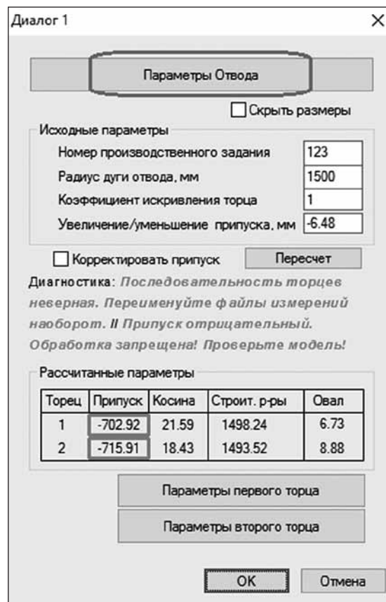
Рис. 5. Диагностика возможности обработки (либо брак заготовки, либо некорректно введенные данные)
