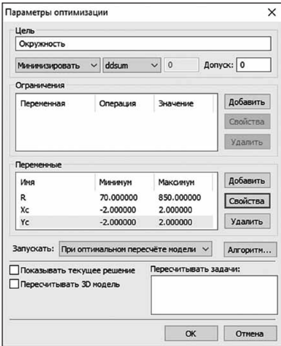
Рис. 2. Задача оптимизации по определению радиуса и центра окружности по облаку точек (измеренных значений), где ddsum – квадратичное отклонение на текущем шаге оптимизации
